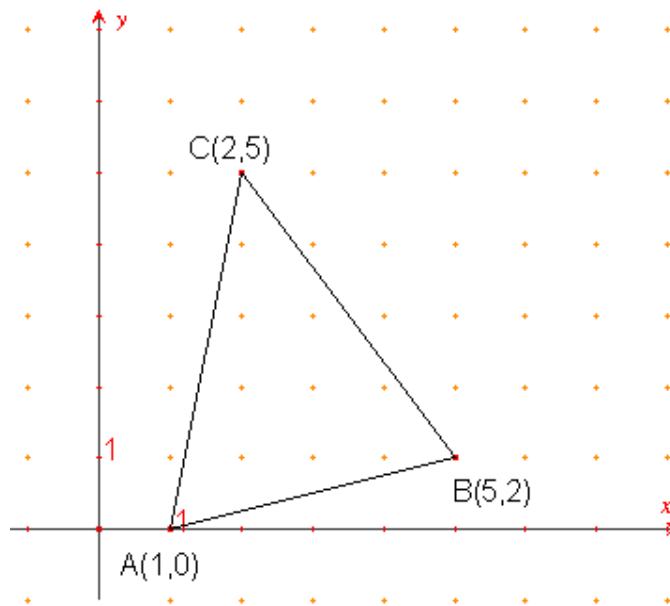
Figura 1: Un triángulo dado.
